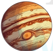
Jupiter
